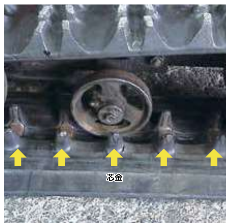
適合芯金タイプクローラ
