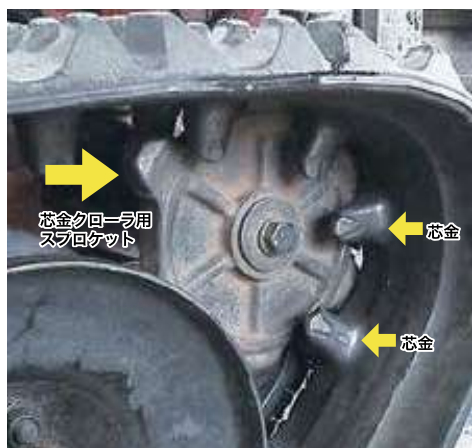
適合芯金タイプクローラ
